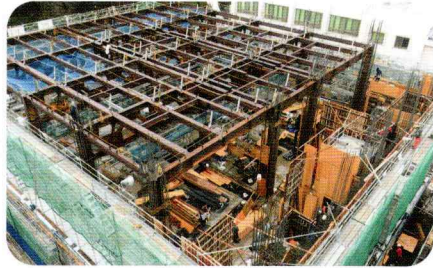
2020年1月 1階鉄骨工事
